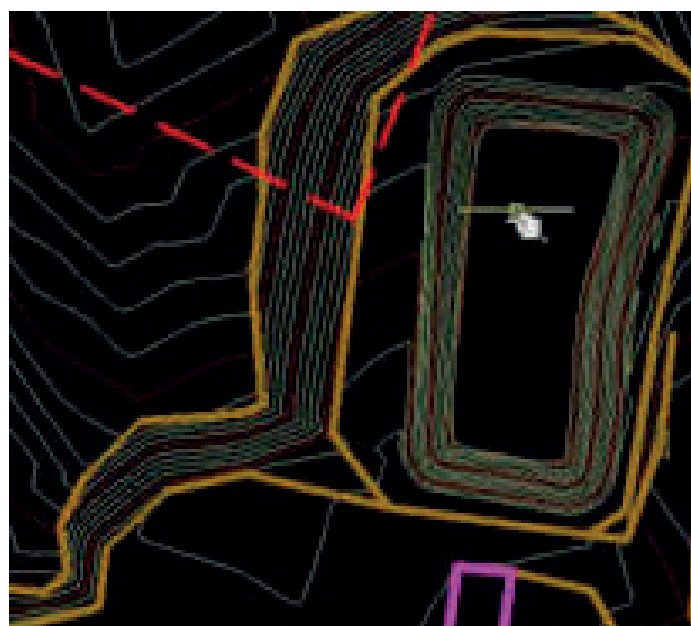
Civil 3D aplicado en proyectos de Minería
